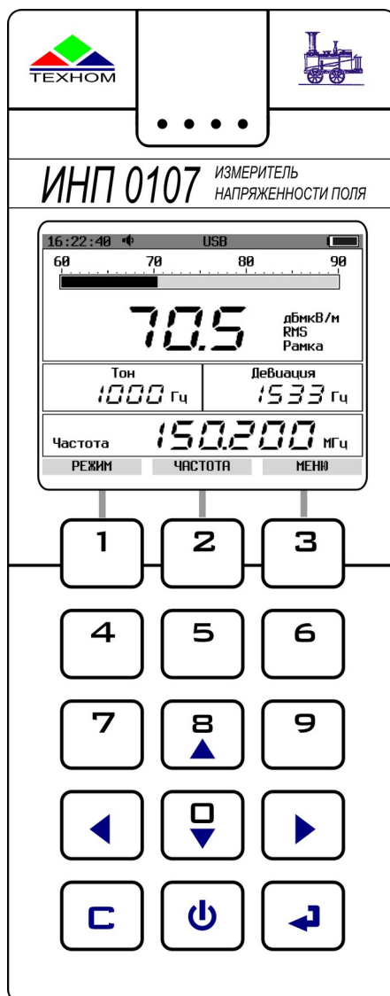
Рис. 1. Лицевая панель индикатора ИНП 0107УКВ
